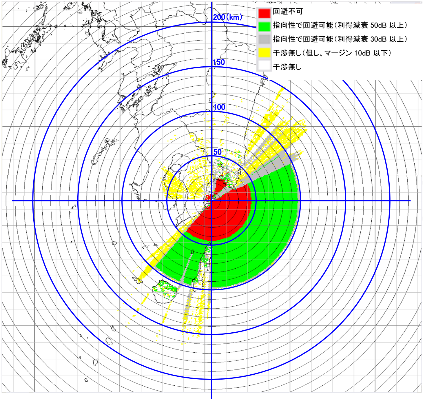
16-① 内之浦 電界強度マップ・・・φ60cm パラボラアンテナ送信機
